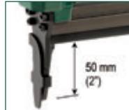
SL változat
